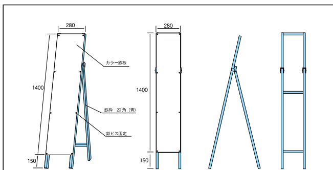
ガードレールスタンド SW-III (スリムタイプ) (AA100-1)
